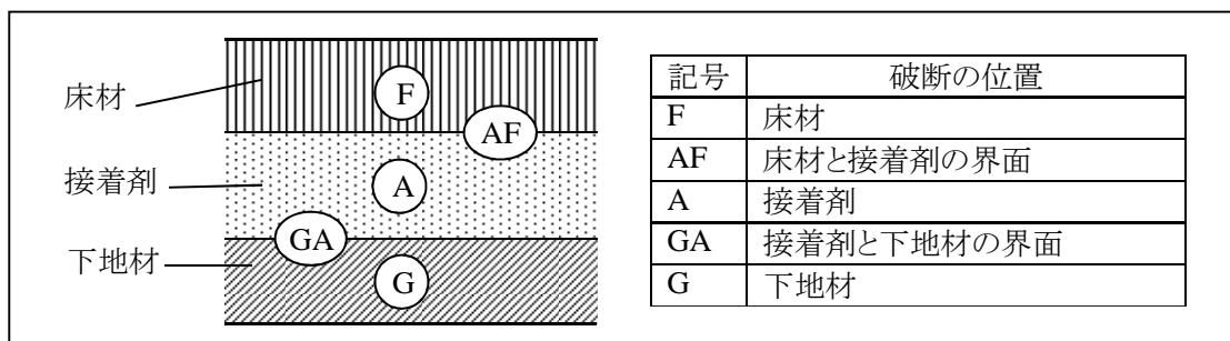
図. 破断の位置及び記号
