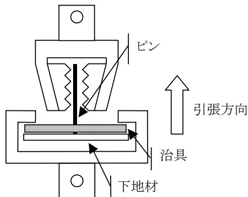
図1:引張試験方法
